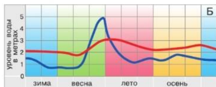
Уровни Волги у г. Ярославля
