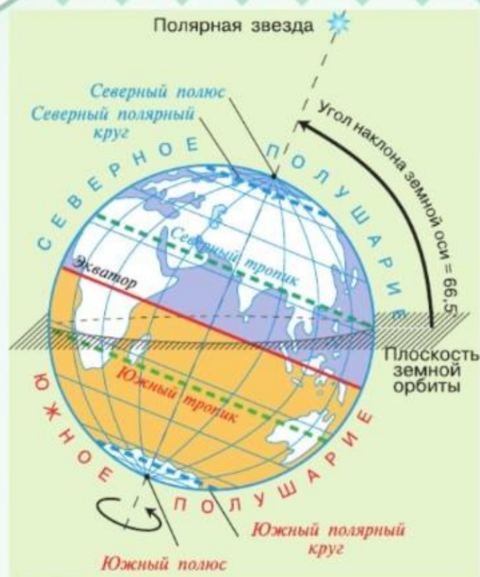
Рис. 26. Схематическое изображение земного шара
