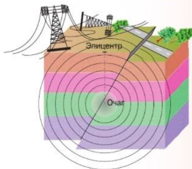
Рис. 57. Схема землетрясения
