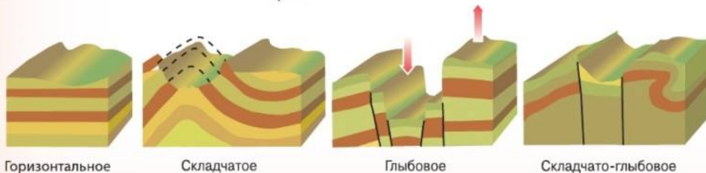
Рис. 56. Схемы залегания горных пород
