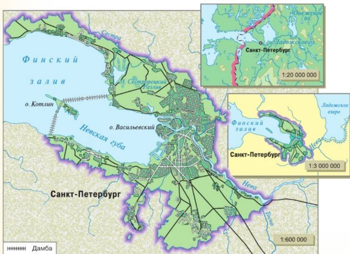
Рис. 41. Территория Санкт-Петербурга в разных масштабах
