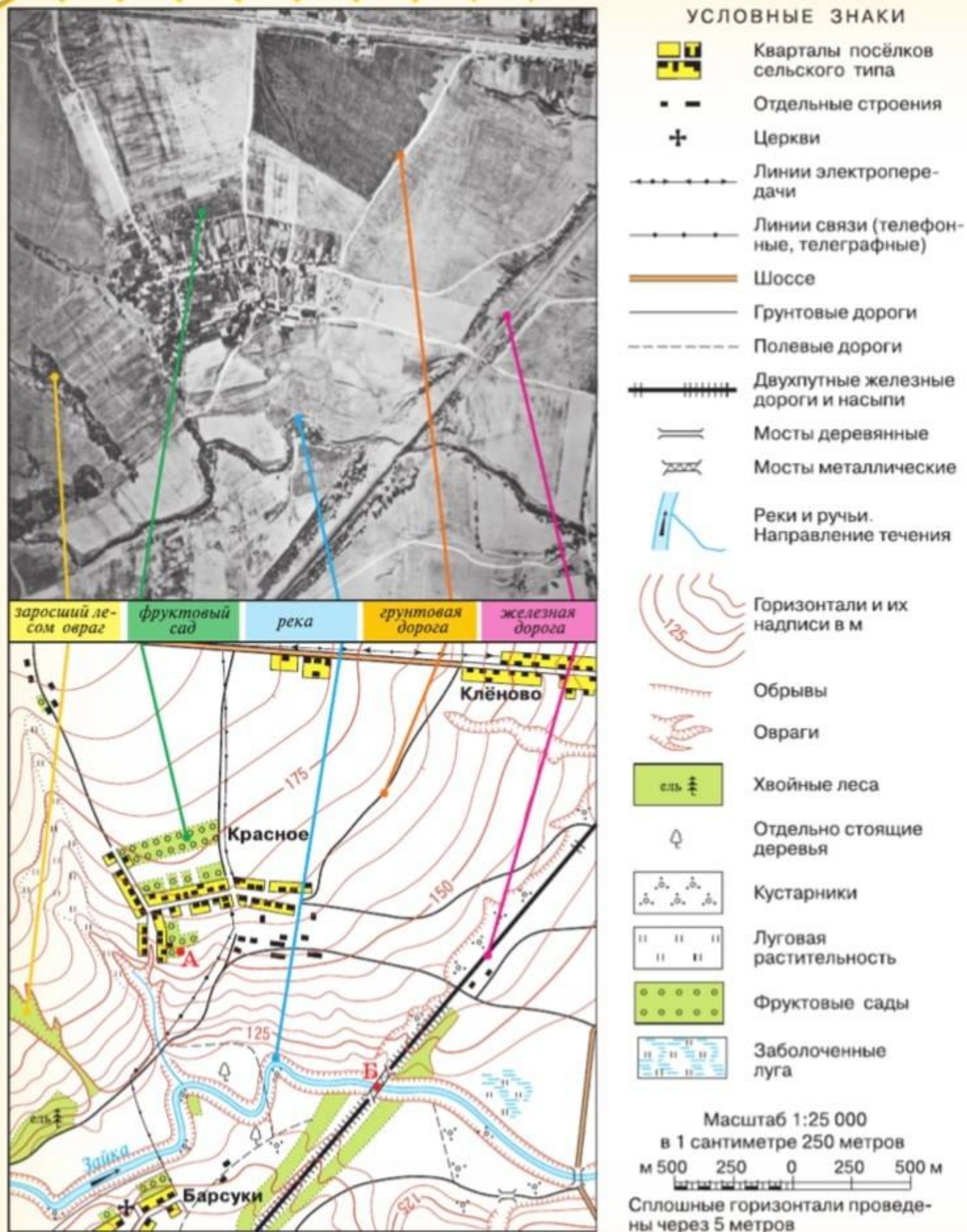
Рис. 35. Аэрофотоснимок и топографическая карта одной и той же местности. Условные знаки
